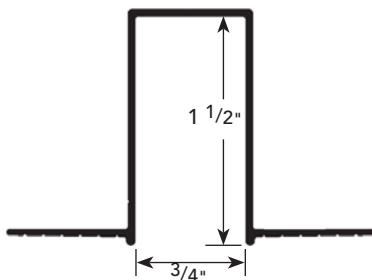
DRYWALL CEILING TRACK (DRM-150-75)
